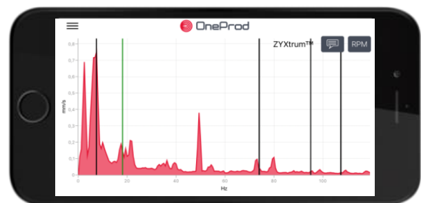
Ejemplo de defecto del rodamiento: una de las frecuencias de falla del rodamiento coincide con un pico en el ZYXtrum™
